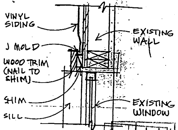
A JAMB
