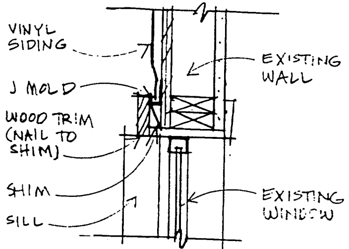
A JAMB
