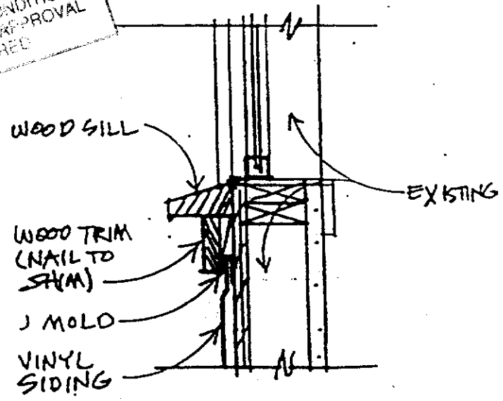
B) SILL
