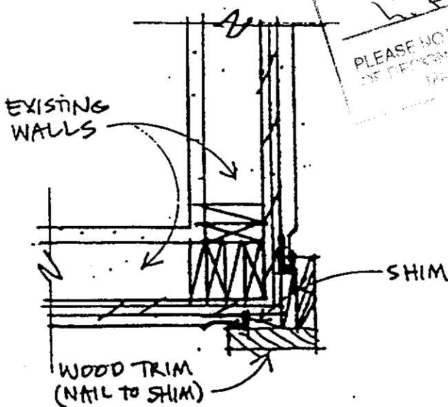
C) CORNER
